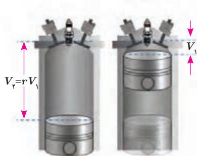
شکل ۱۷-۵ حجم فضای بالای پیستون در ابتدا V_1 و در انتها rV_1 است.
