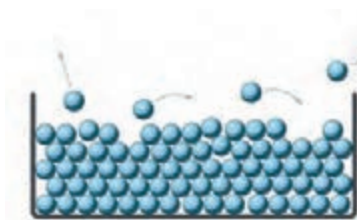
شکل ۴-۲۳ در حین تبخیر سطحی، مولکول‌های پیرانزی تر از سطح مایع می‌گریزند.
