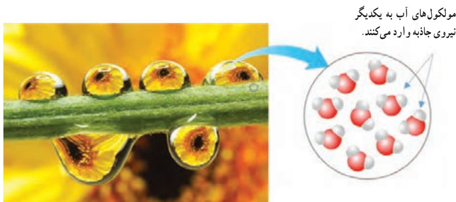
شکل ۷-۲ قطره‌های شبی که روی شاخ و برگ درختان در نور خورشید صبحگاهی می‌درخشند، نشانه‌ای از نیروی جاذبه بین مولکول‌های آب است.
